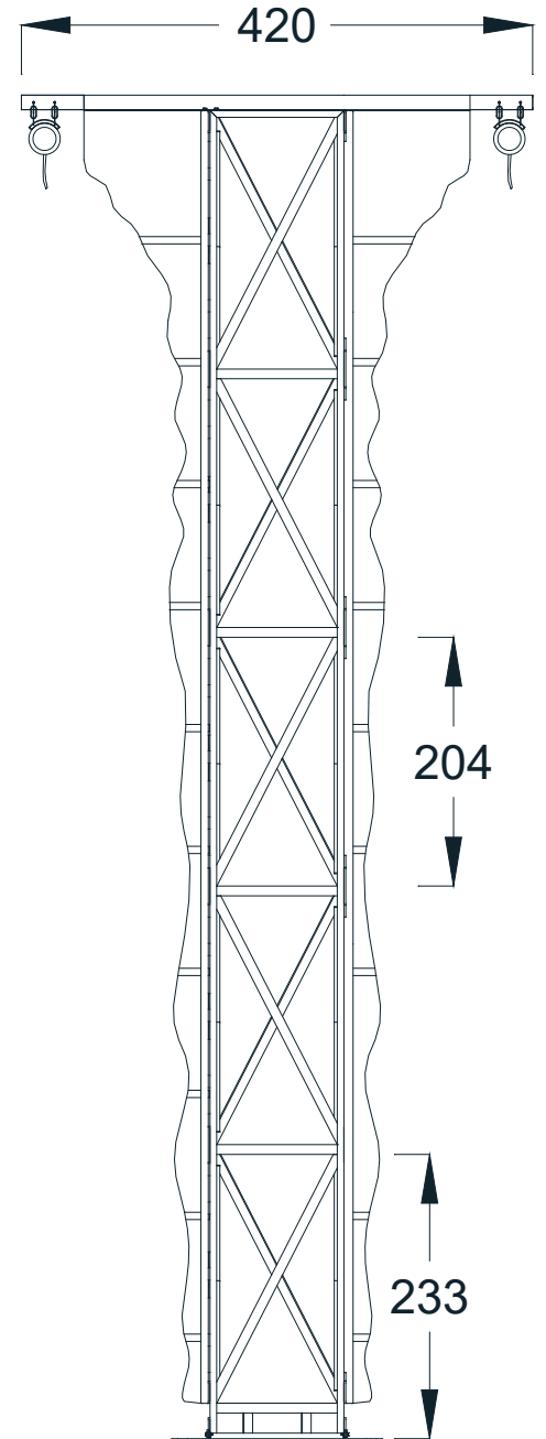
YAN GÖRÜNÜŞ / SIDE VIEW
