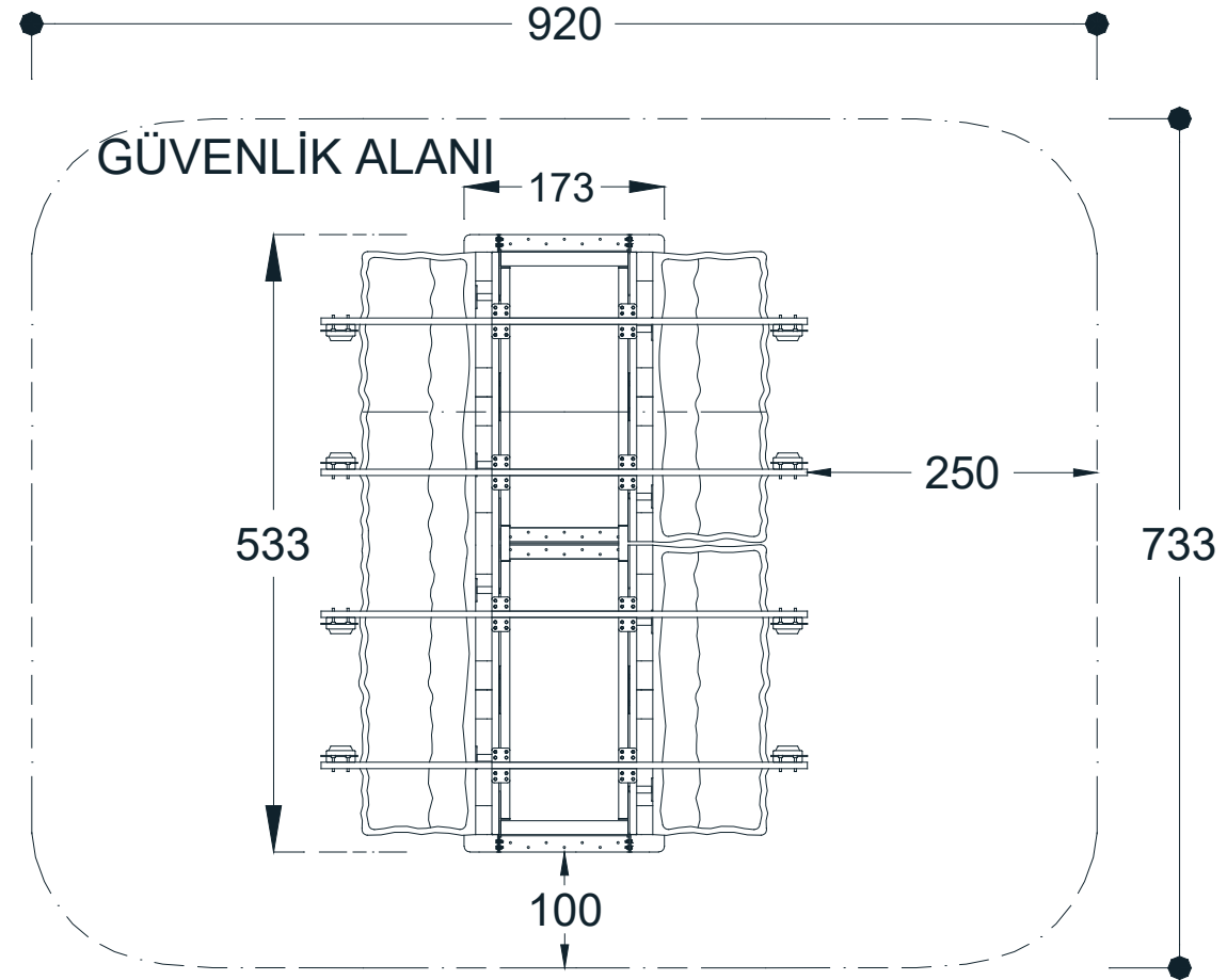
ÜST GÖRÜNÜŞ / TOP VIEW
