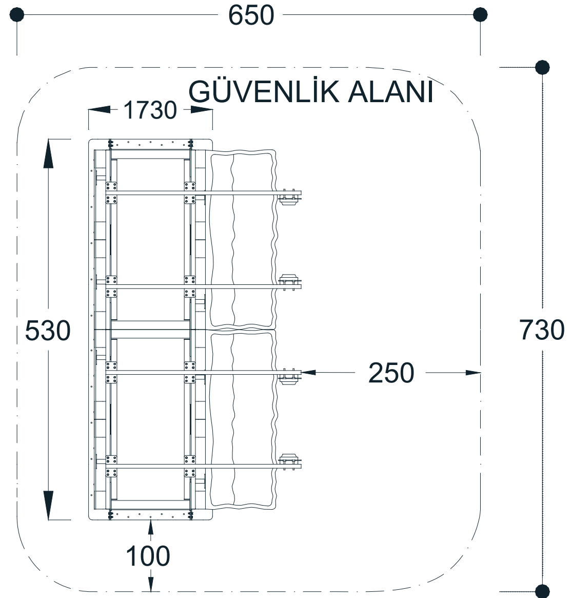
ÜST GÖRÜNÜŞ / TOP VIEW
