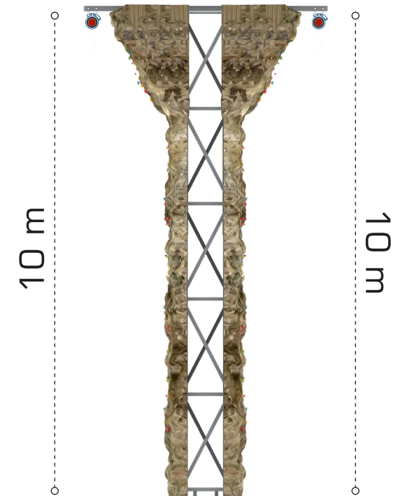
YAN GÖRÜNÜŞ / SIDE VIEW
