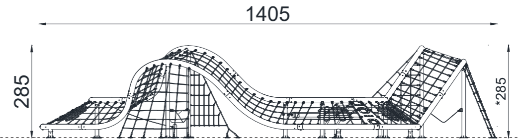
YAN GÖRÜNÜŞ / SIDE VIEW
