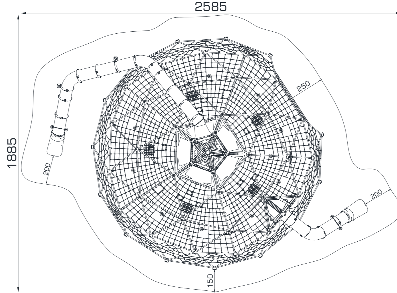
ÜST GÖRÜNÜŞ / TOP VIEW
