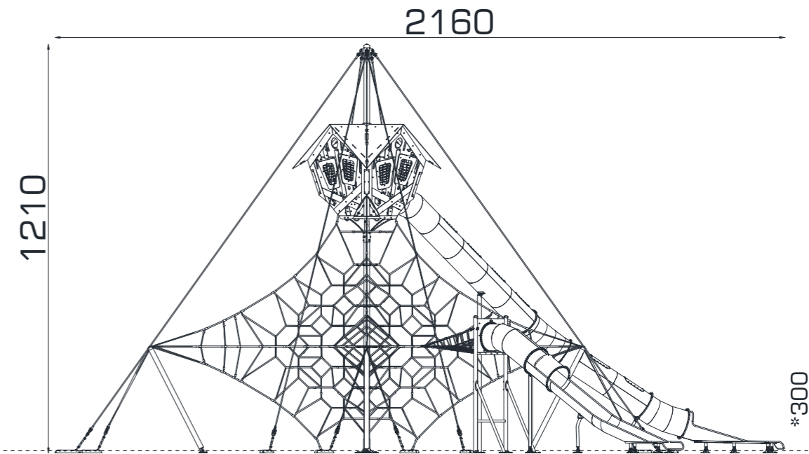
YAN GÖRÜNÜŞ / SIDE VIEW
