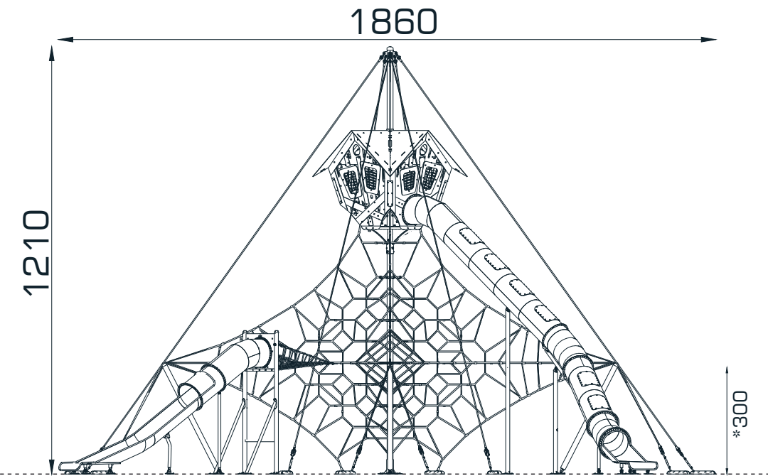
YAN GÖRÜNÜŞ / SIDE VIEW
