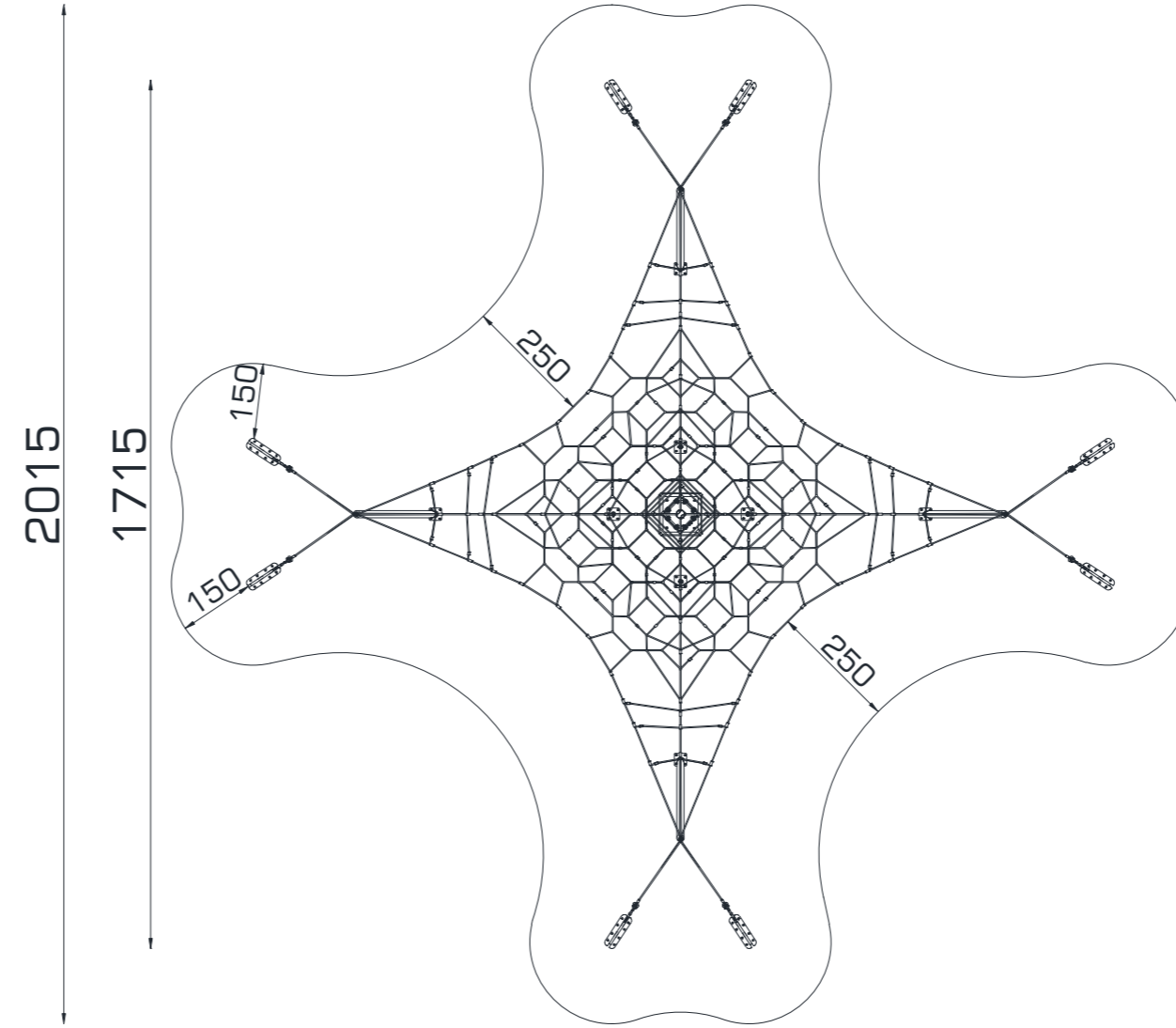
ÜST GÖRÜNÜŞ / TOP VIEW
