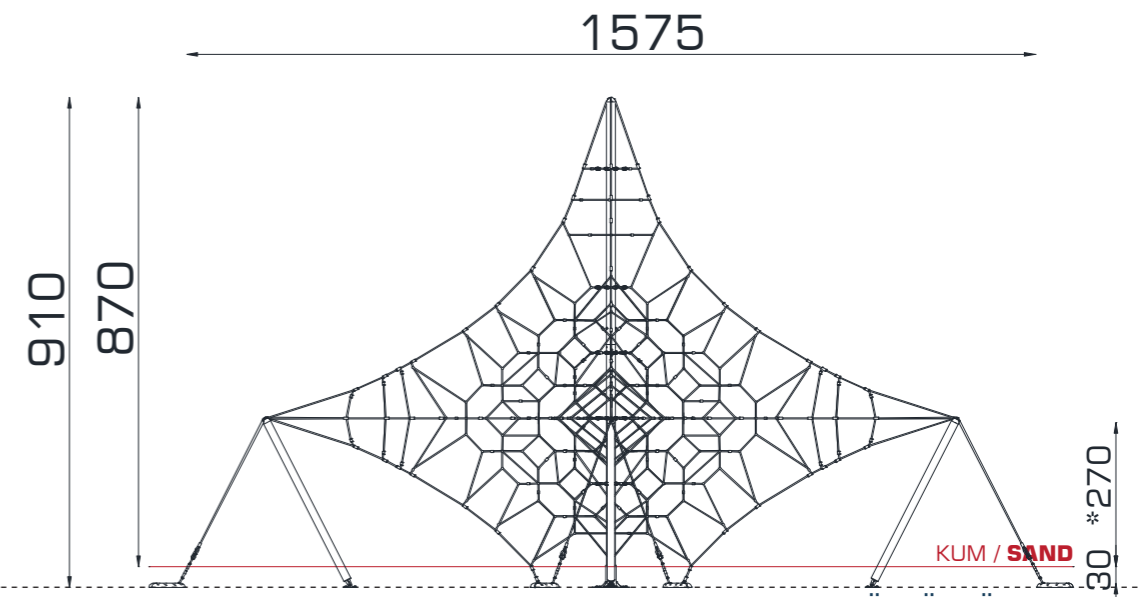
YAN GÖRÜNÜŞ / SIDE VIEW
