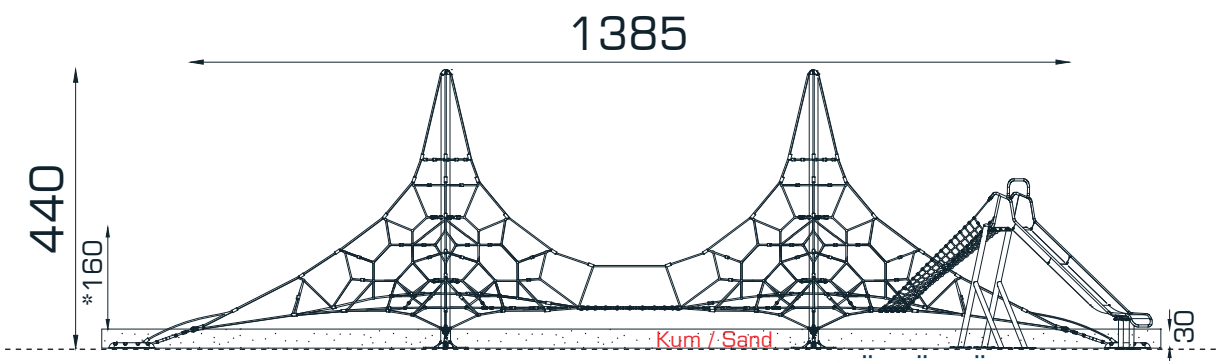
YAN GÖRÜNÜŞ / SIDE VIEW
