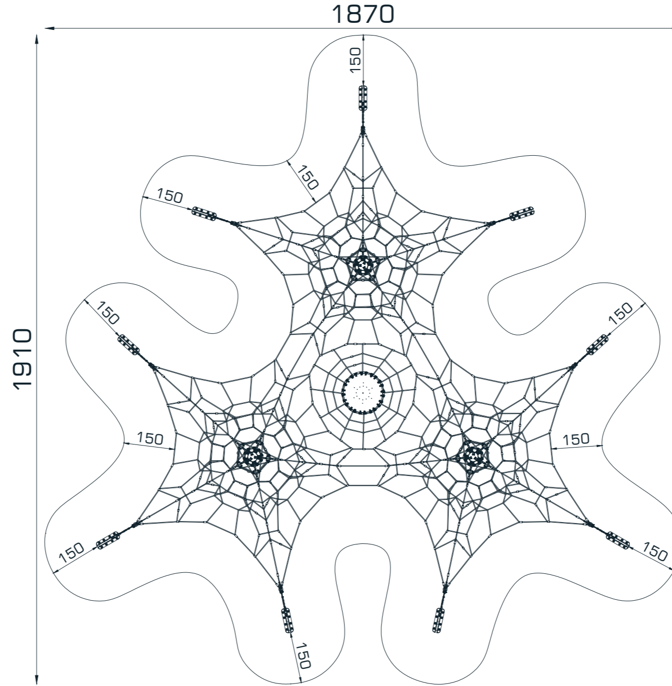
ÜST GÖRÜNÜŞ / TOP VIEW
