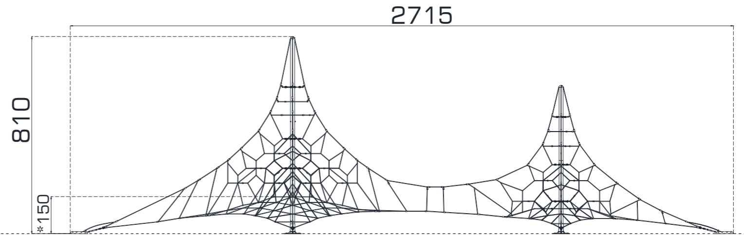
YAN GÖRÜNÜŞ / SIDE VIEW
