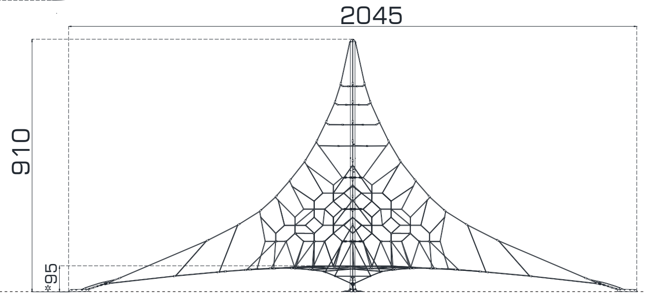
YAN GÖRÜNÜŞ / SIDE VIEW
