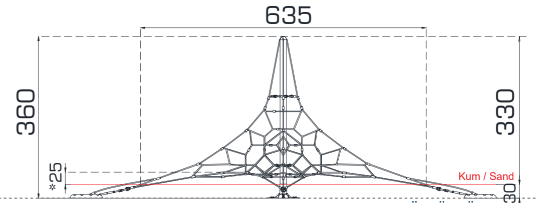
YAN GÖRÜNÜŞ / SIDE VIEW
