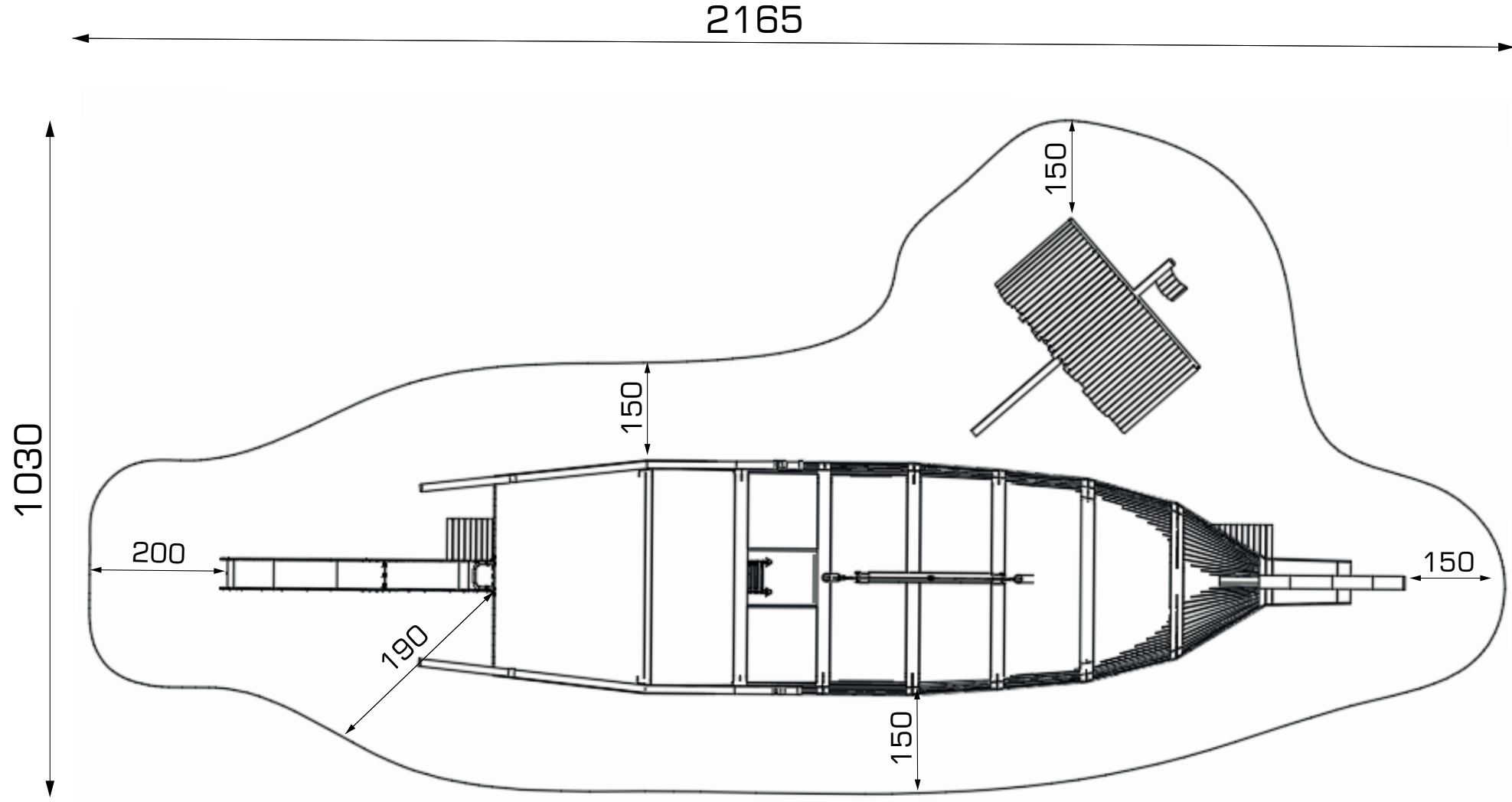
ÜST GÖRÜNÜŞ / TOP VIEW
