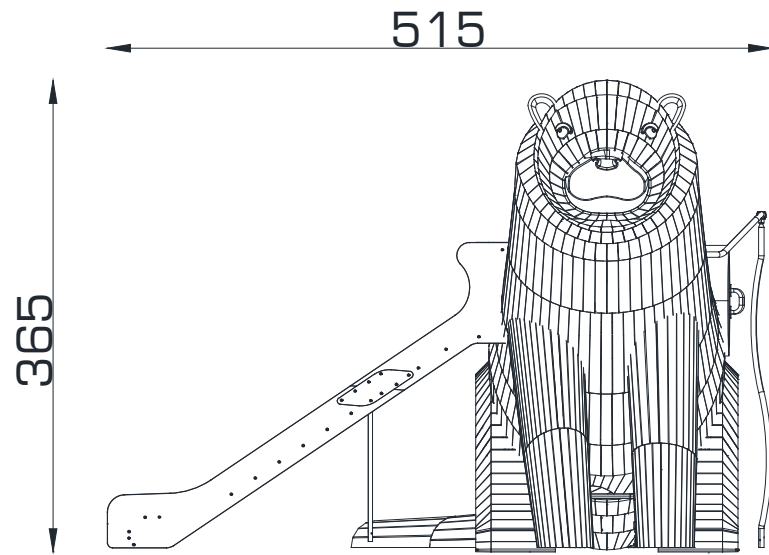
ÖN GÖRÜNÜŞ / FRONT VIEW
