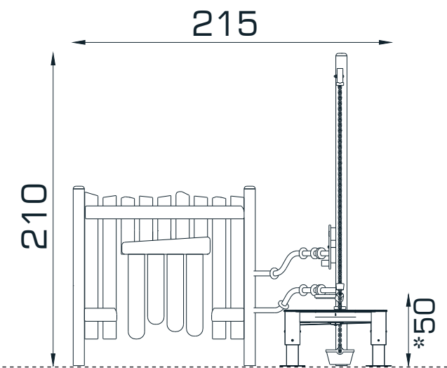
YAN GÖRÜNÜŞ / SIDE VIEW
