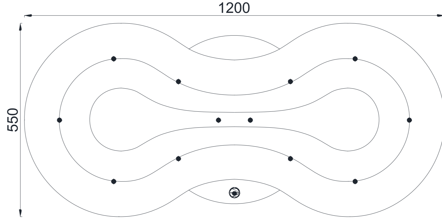
ÜST GÖRÜNÜŞ / TOP VIEW
