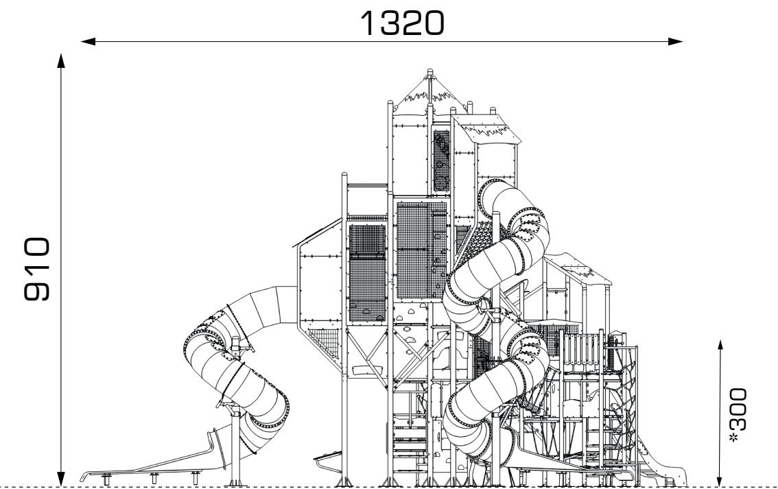
YAN GÖRÜNÜŞ / SIDE VIEW
