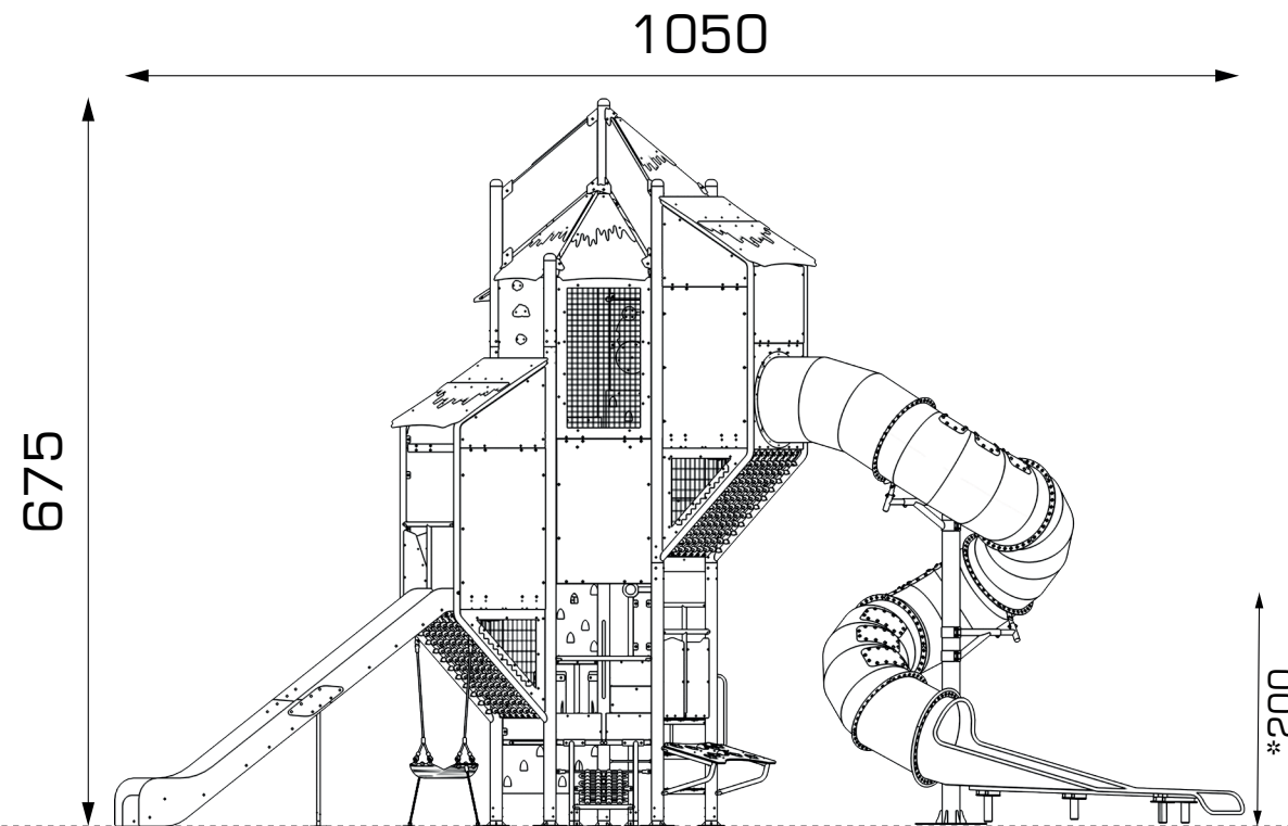
ÖN GÖRÜNÜŞ / FRONT VIEW
