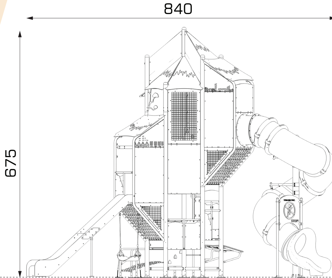
ÖN GÖRÜNÜŞ / FRONT VIEW
