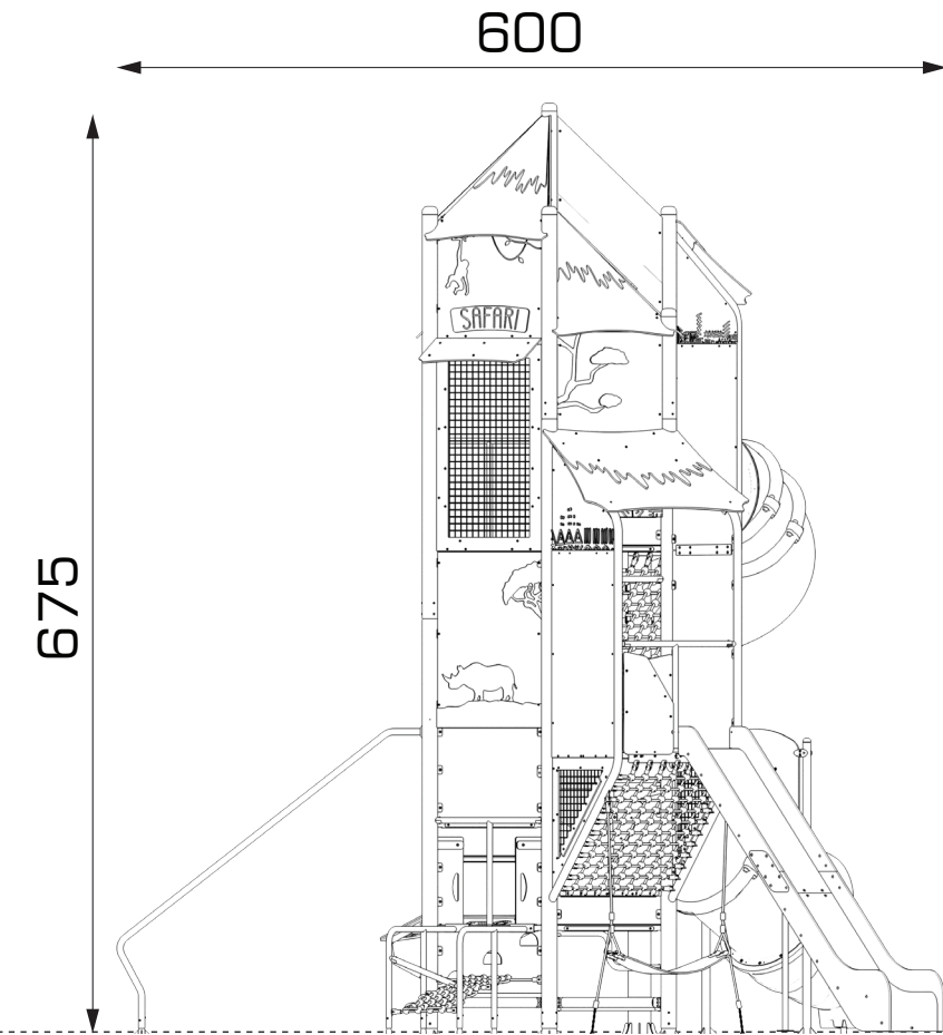
YAN GÖRÜNÜŞ / SIDE VIEW
