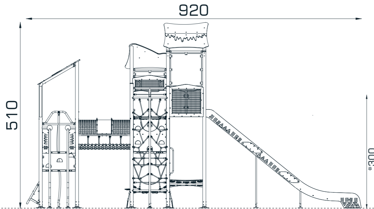
ÖN GÖRÜNÜŞ / FRONT VIEW
