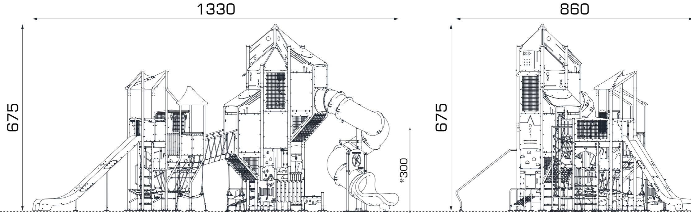
ÖN GÖRÜNÜŞ / FRONT VIEW
