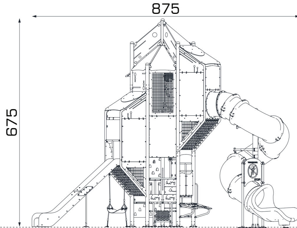
ÖN GÖRÜNÜŞ / FRONT VIEW
