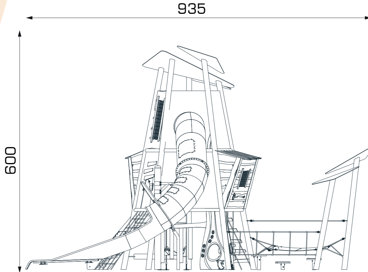
ÖN GÖRÜNÜŞ / FRONT VIEW
