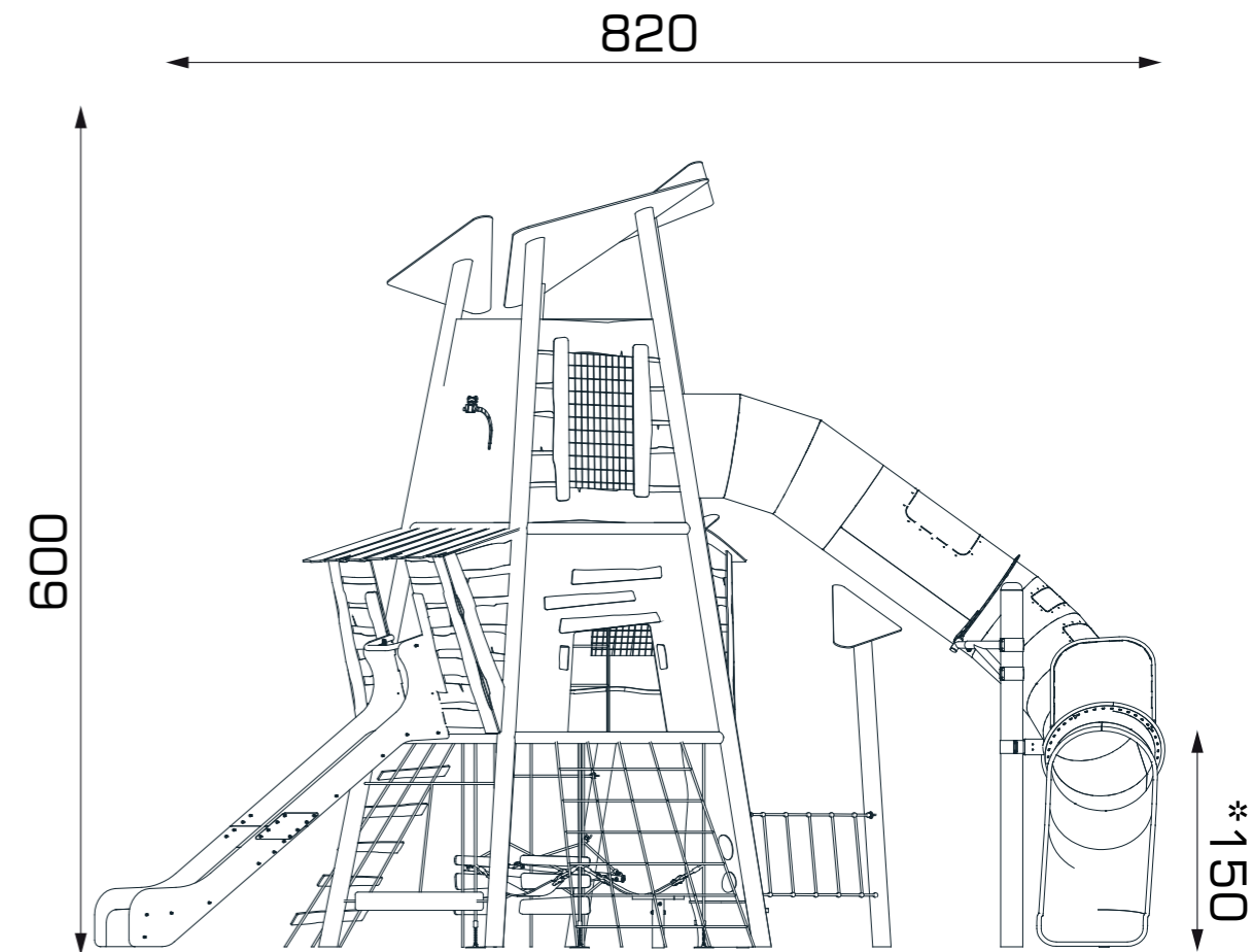
YAN GÖRÜNÜŞ / SIDE VIEW
