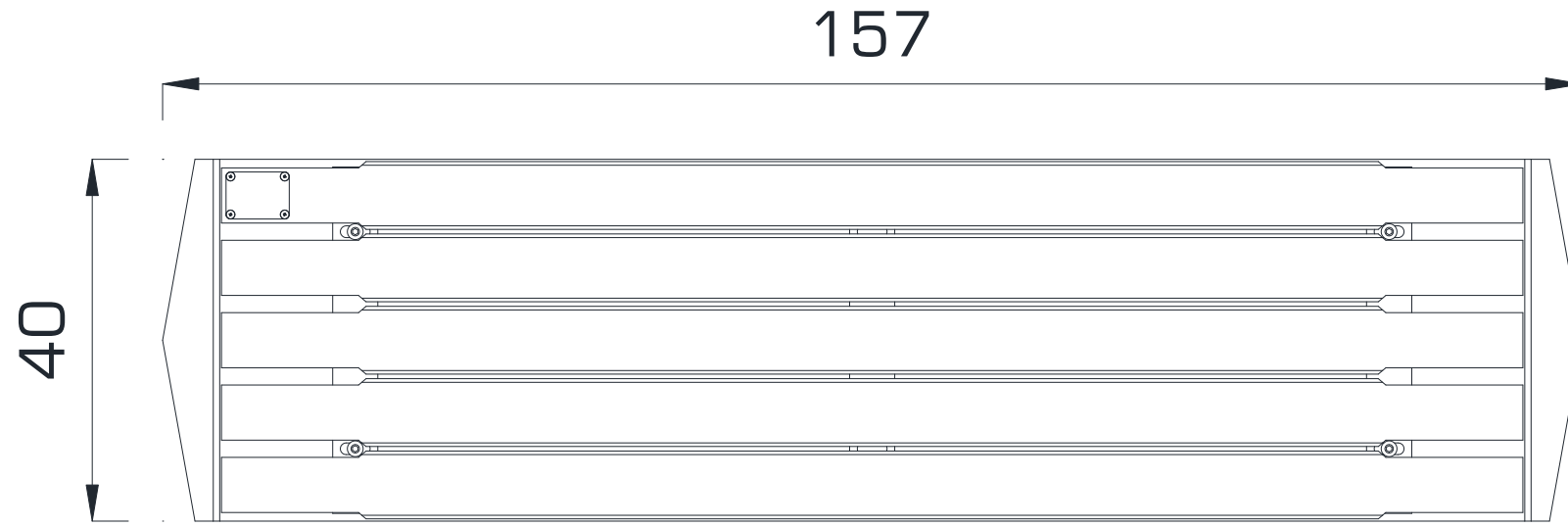
ÜST GÖRÜNÜŞ / TOP VIEW
