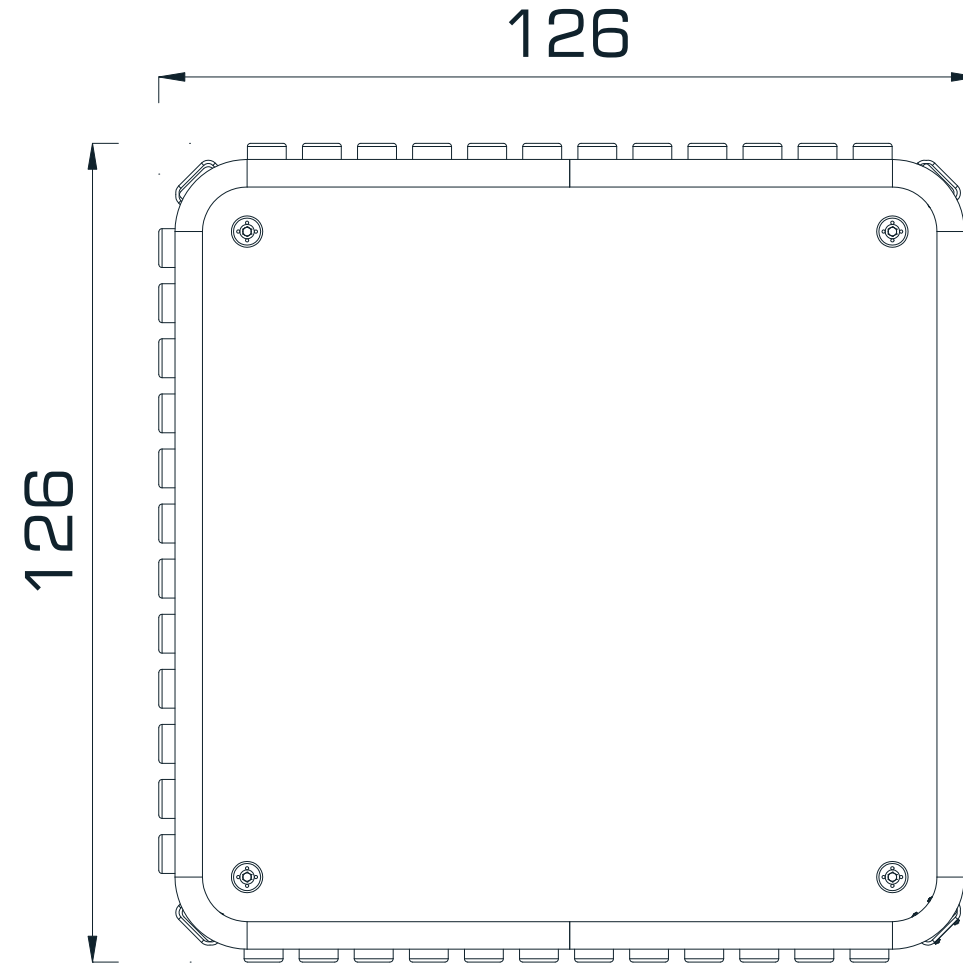
ÜST GÖRÜNÜŞ / TOP VIEW
