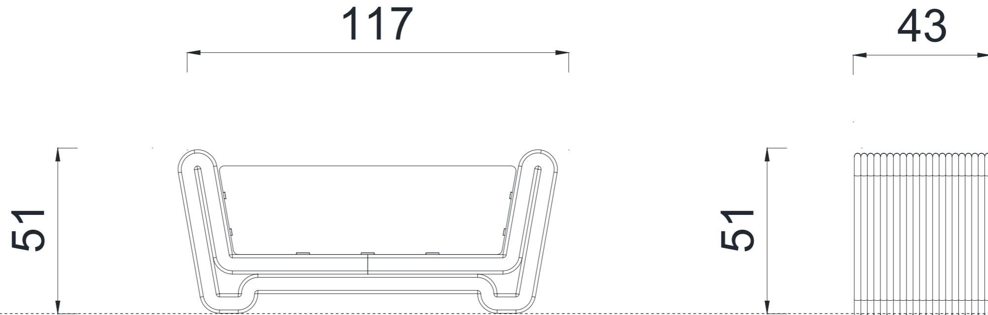
ÖN GÖRÜNÜŞ / FRONT VIEW
