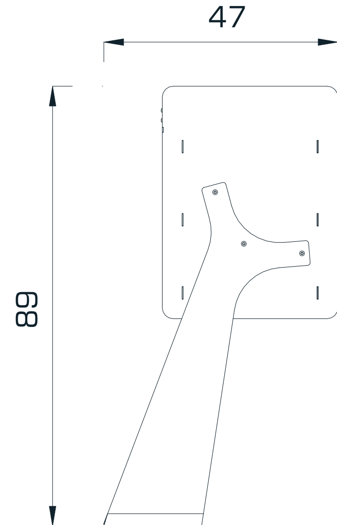
YAN GÖRÜNÜŞ / SIDE VIEW
