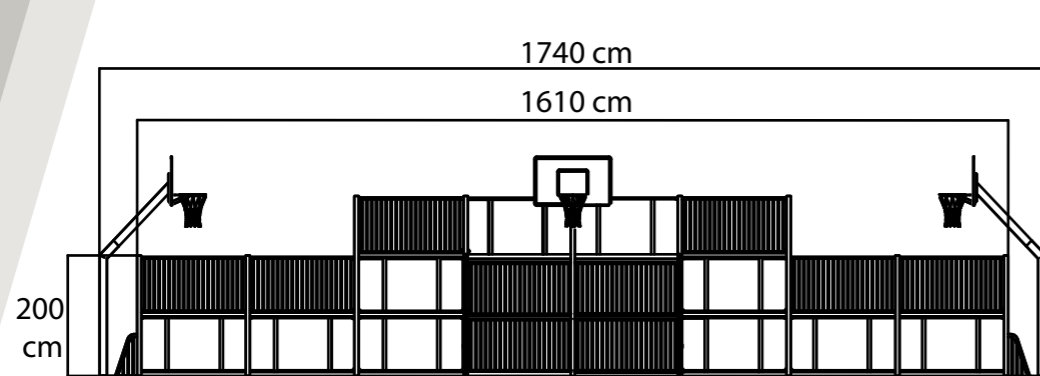
ÖN GÖRÜNÜŞ / FRONT VIEW
