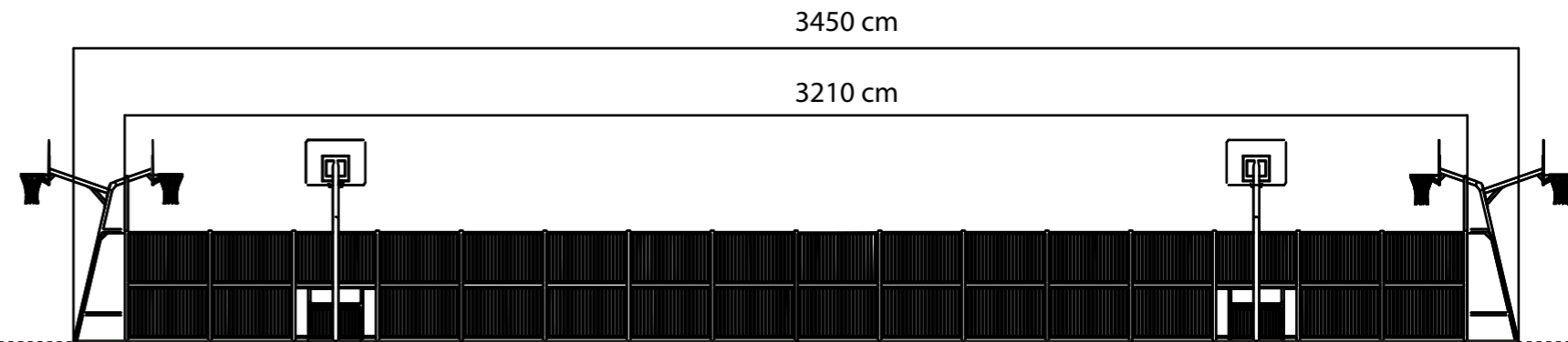
YAN GÖRÜNÜŞ / SIDE VIEW
