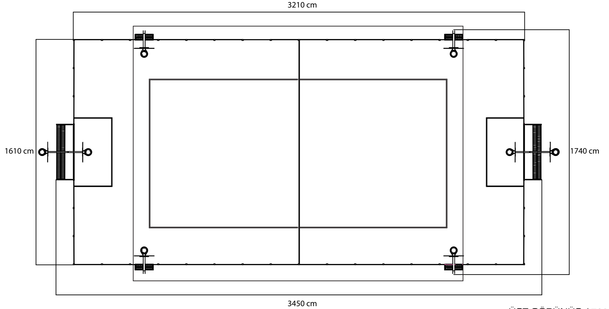
ÜST GÖRÜNÜŞ / TOP VIEW
