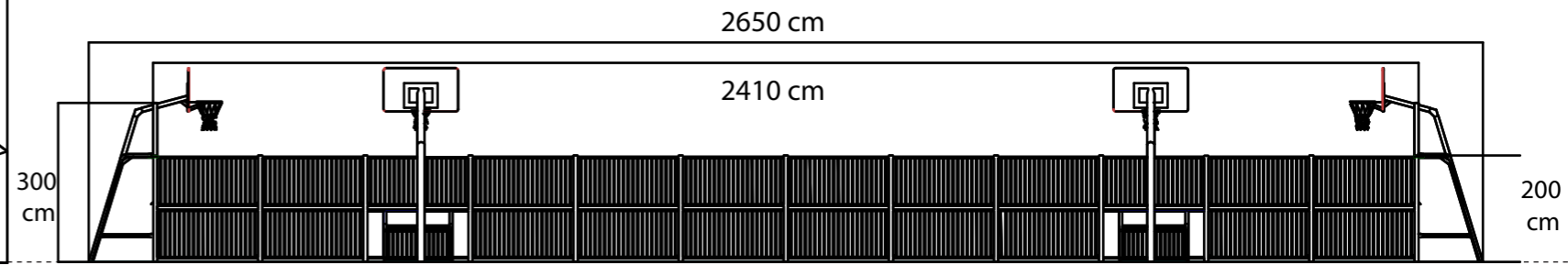
YAN GÖRÜNÜŞ / SIDE VIEW
