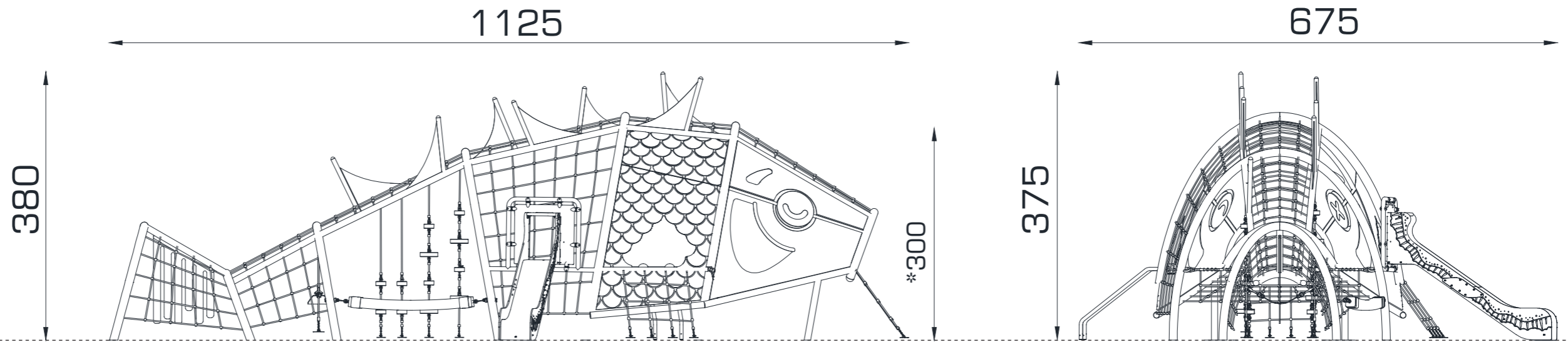
ÖN GÖRÜNÜŞ / FRONT VIEW
