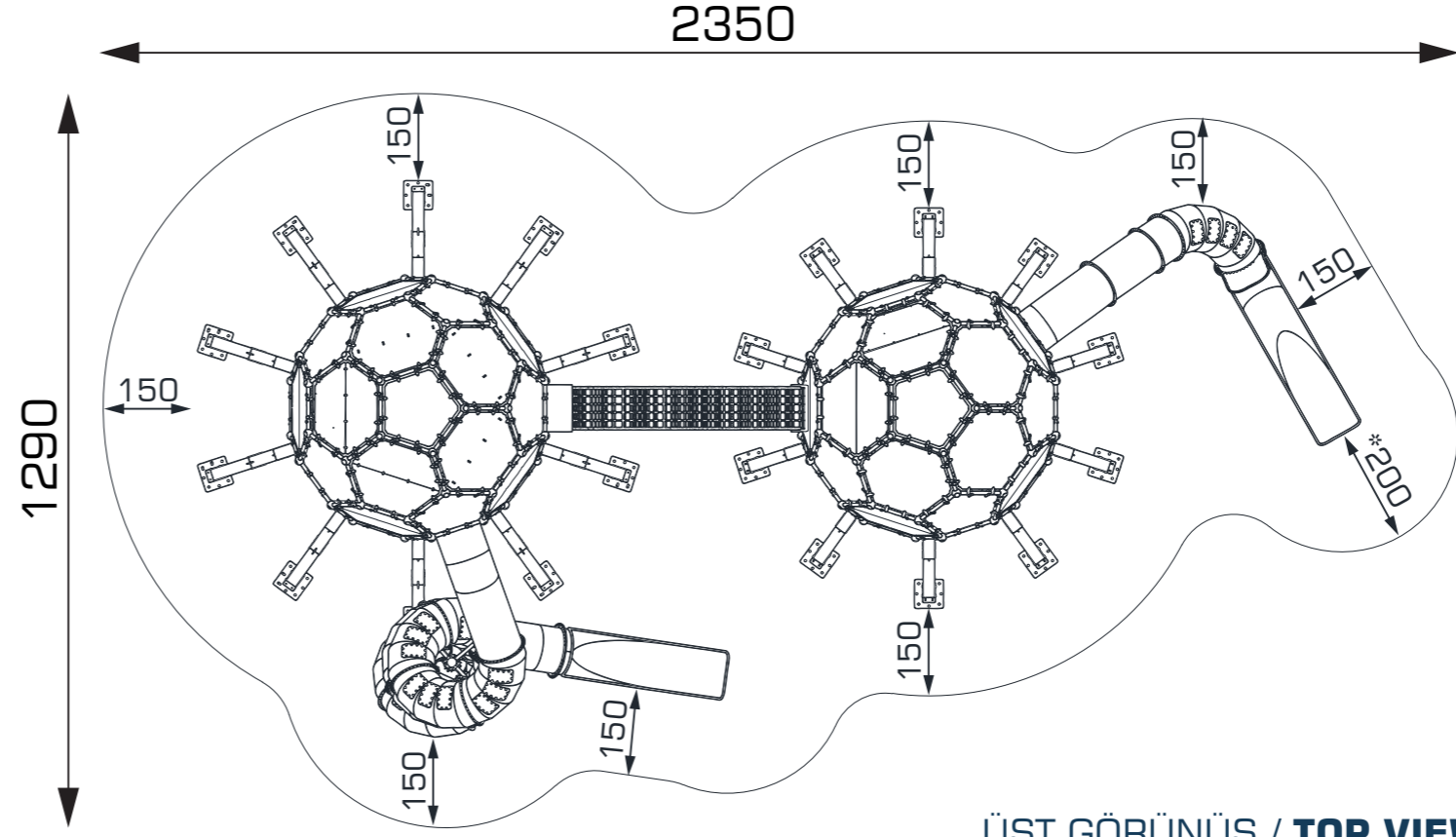
ÜST GÖRÜNÜŞ / TOP VIEW
