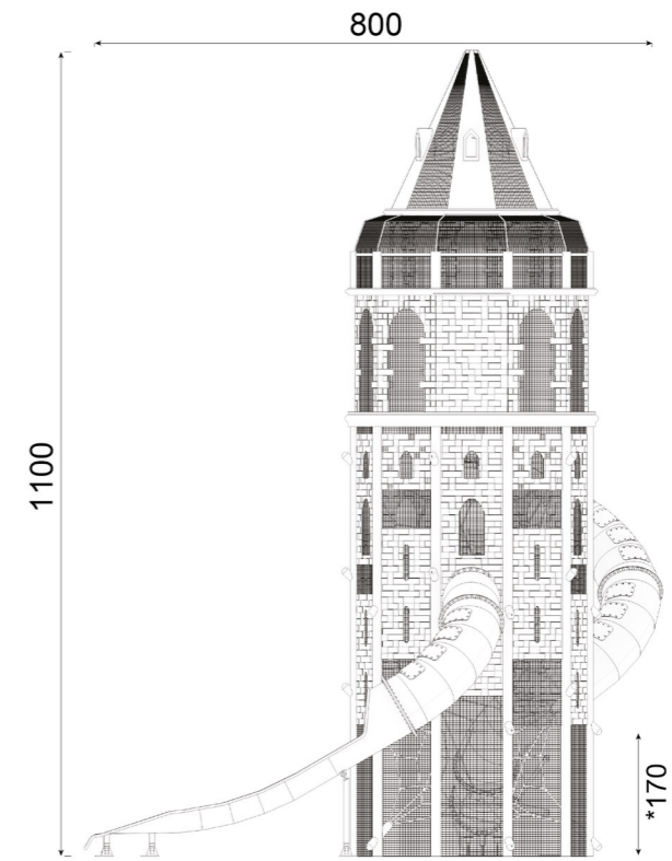
YAN GÖRÜNÜŞ / SIDE VIEW
