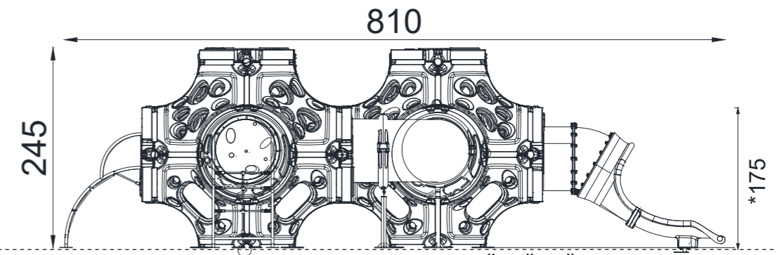
YAN GÖRÜNÜŞ / SIDE VIEW
