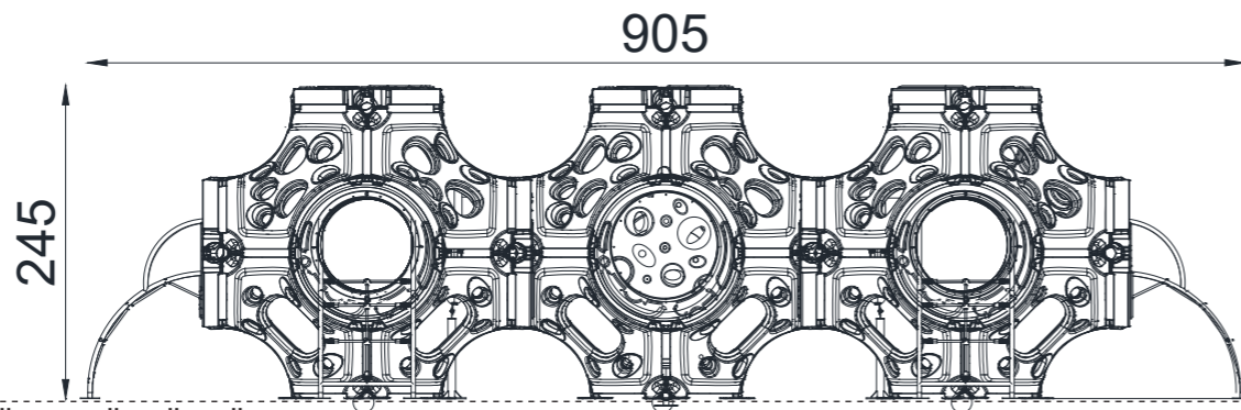
ÖN GÖRÜNÜŞ / FRONT VIEW
