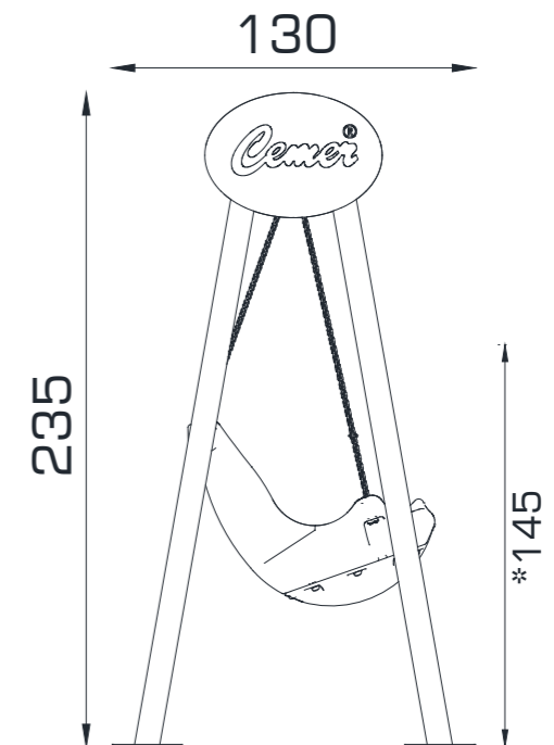
YAN GÖRÜNÜŞ / SIDE VIEW
