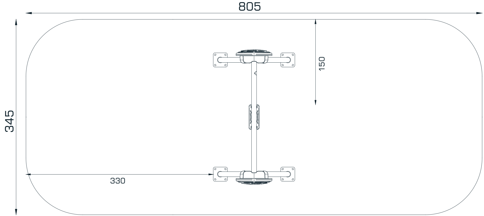
ÜST GÖRÜNÜŞ / TOP VIEW
