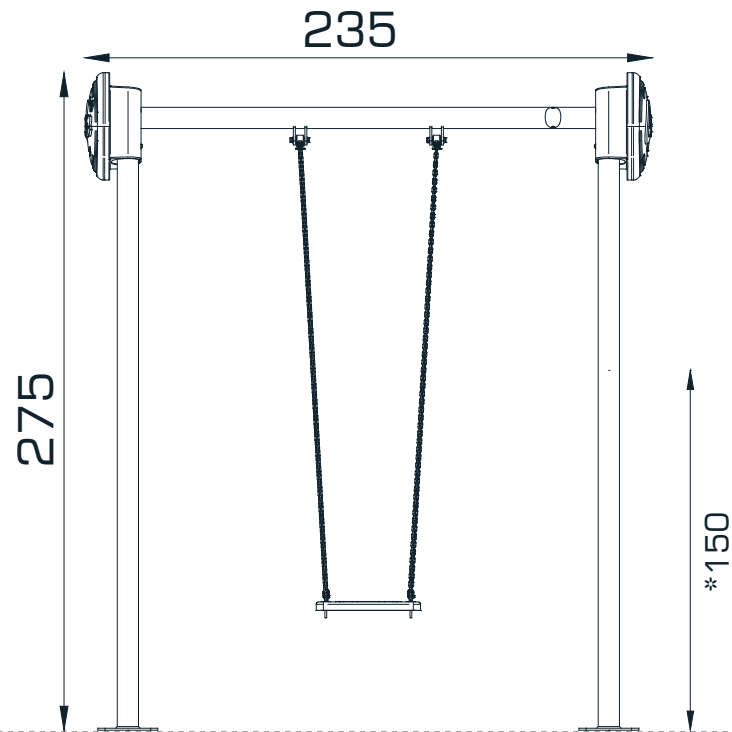
ÖN GÖRÜNÜŞ / FRONT VIEW
