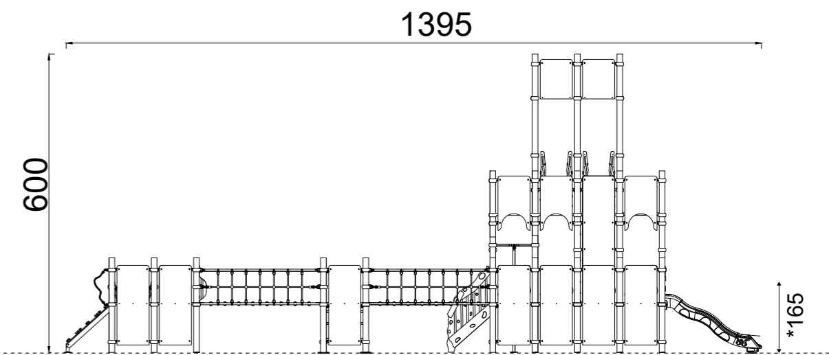
YAN GÖRÜNÜŞ / SIDE VIEW
