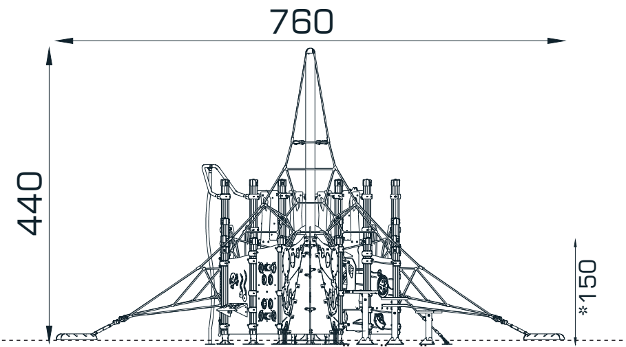
YAN GÖRÜNÜŞ / SIDE VIEW
