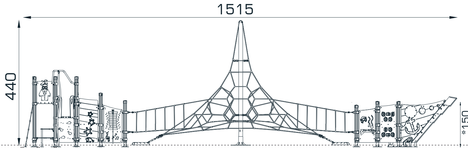
ÖN GÖRÜNÜŞ / FRONT VIEW
