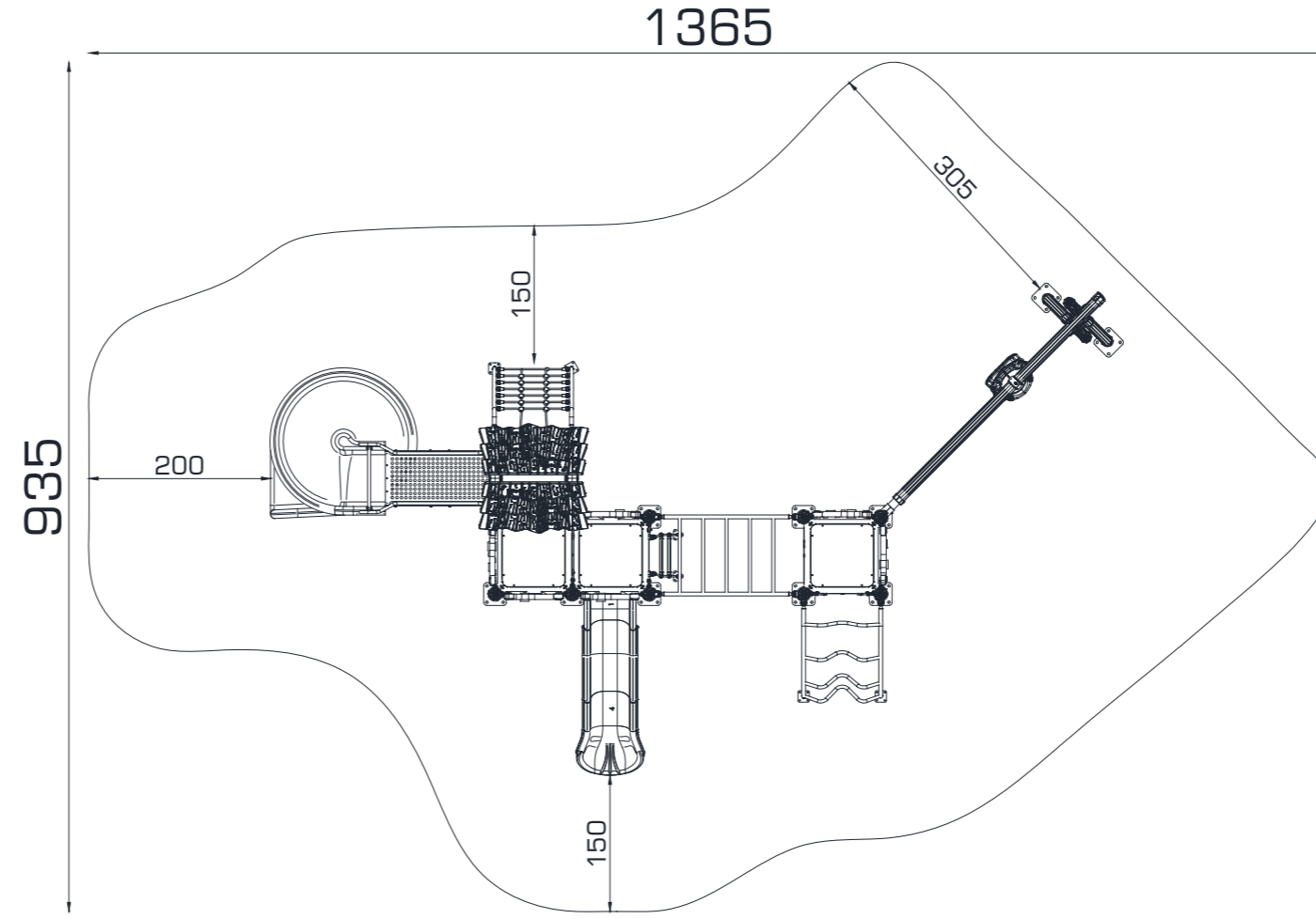
ÜST GÖRÜNÜŞ / TOP VIEW
