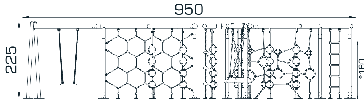
ÖN GÖRÜNÜŞ / FRONT VIEW
