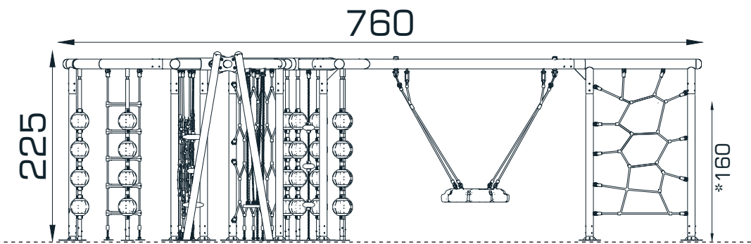
YAN GÖRÜNÜŞ / SIDE VIEW
