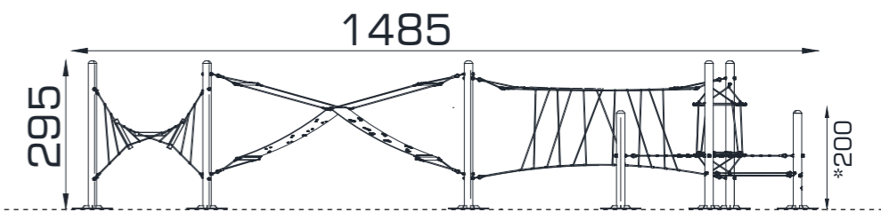
YAN GÖRÜNÜŞ / SIDE VIEW
