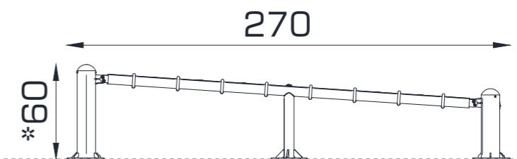
YAN GÖRÜNÜŞ / SIDE VIEW
