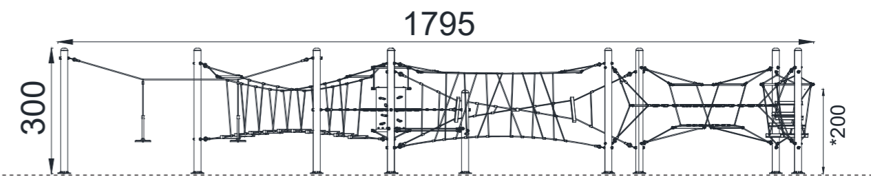
YAN GÖRÜNÜŞ / SIDE VIEW
