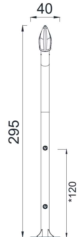
YAN GÖRÜNÜŞ / SIDE VIEW
