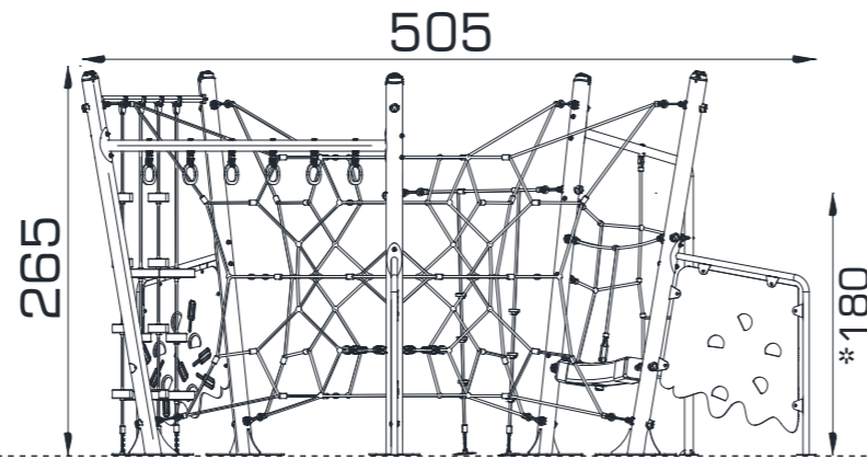
ÖN GÖRÜNÜŞ / FRONT VIEW
