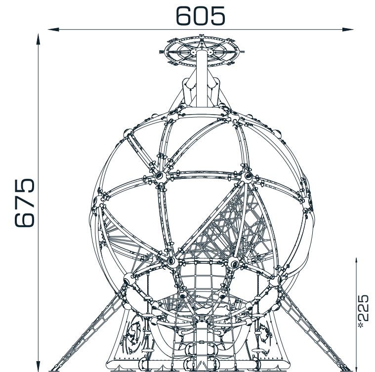
YAN GÖRÜNÜŞ / SIDE VIEW
