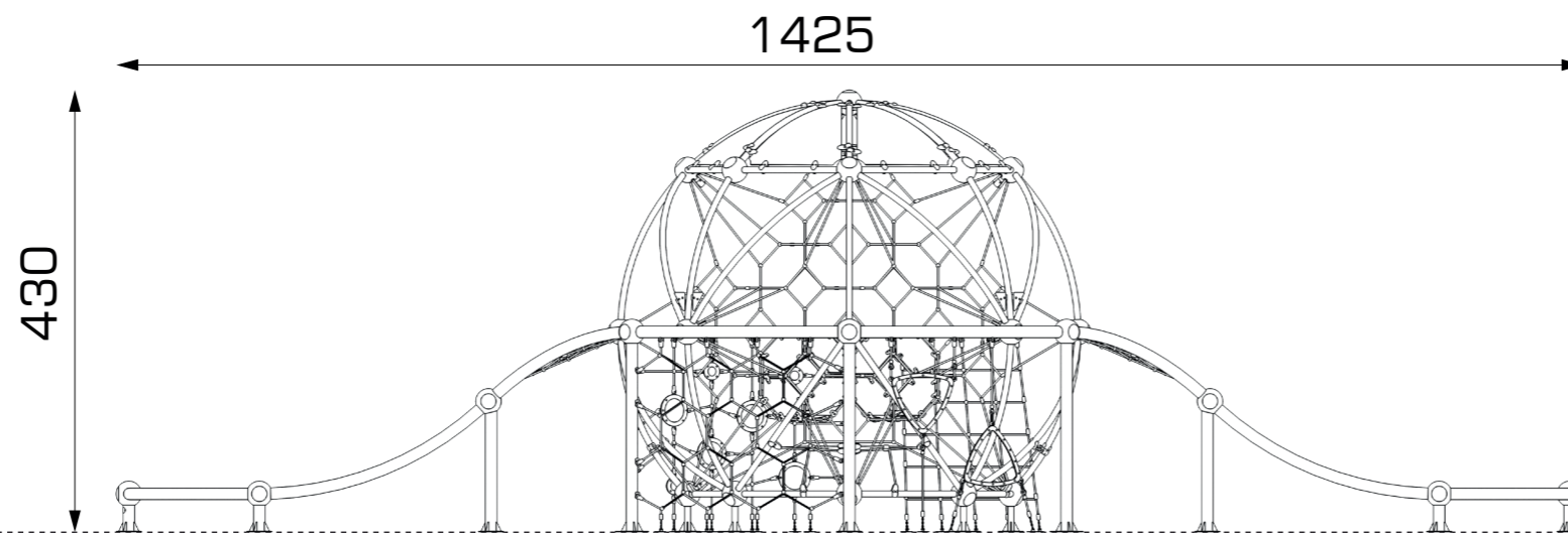
ÖN GÖRÜNÜŞ / FRONT VIEW
