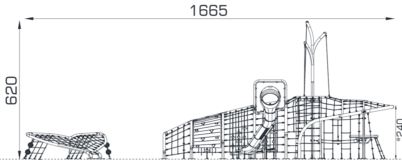
ÖN GÖRÜNÜŞ / FRONT VIEW
