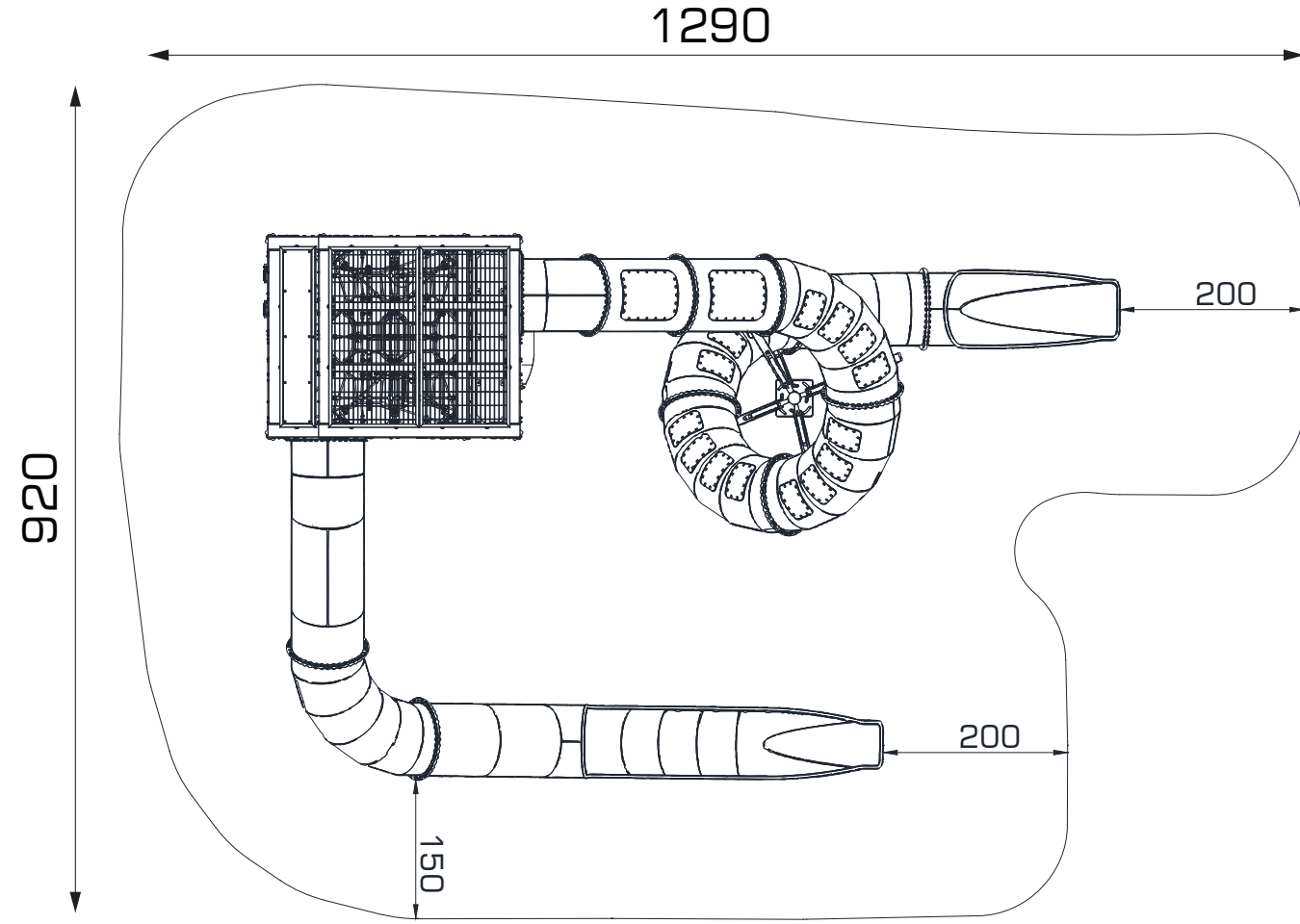
ÜST GÖRÜNÜŞ / TOP VIEW
